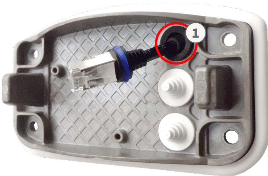
Abb. 22: Montageplatte vorbereiten
